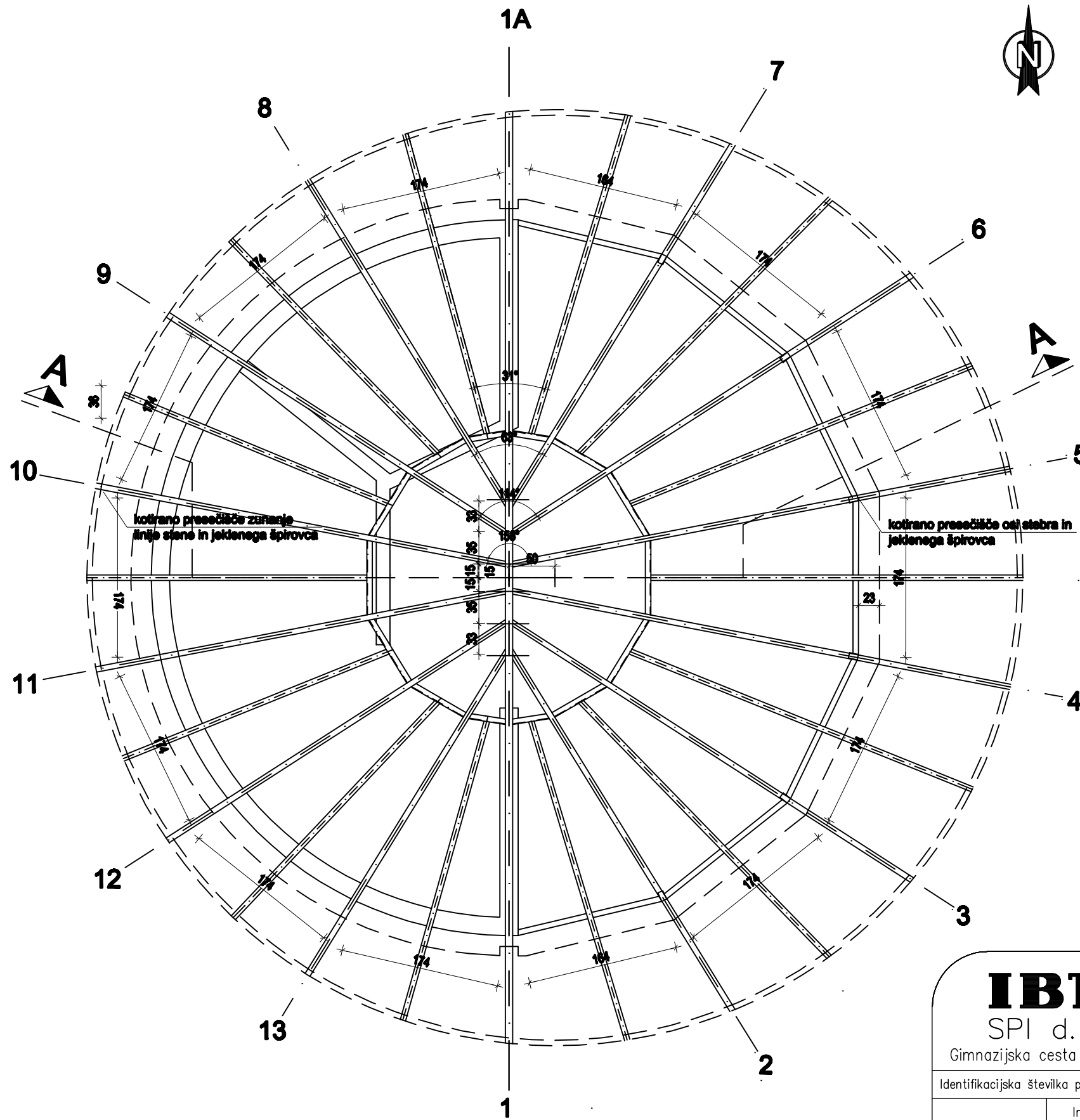
GLEJ OPOMBE NA RISBI TEMELJEV, 1.5.02 Dolžine elementov jeklene konstrukcije ostrešja - načrt gradbenih konstrukcij - risba delavniški načrt - št.3
